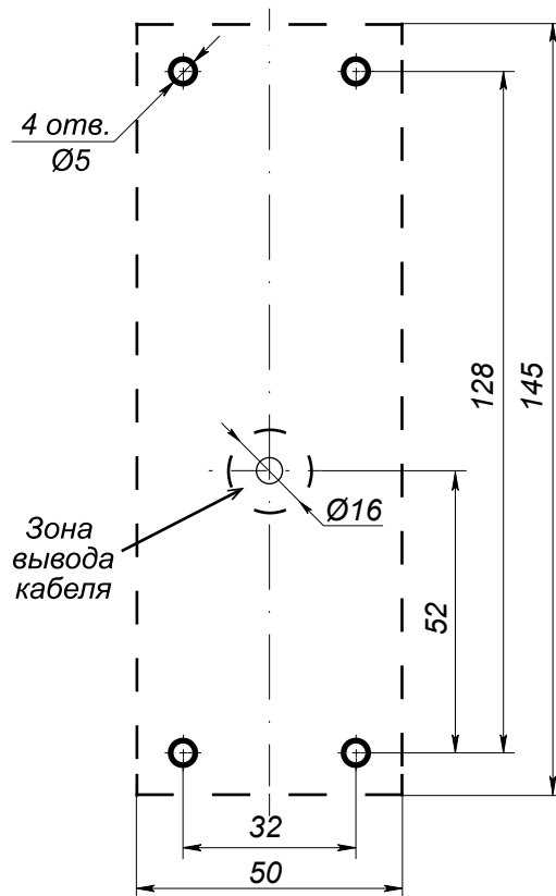
Разметка отверстий для установки считывателя
