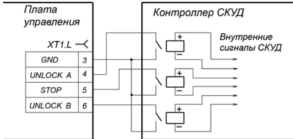
Рисунок 5. Управляющий элемент СКУД – нормально разомкнутый контакт реле
