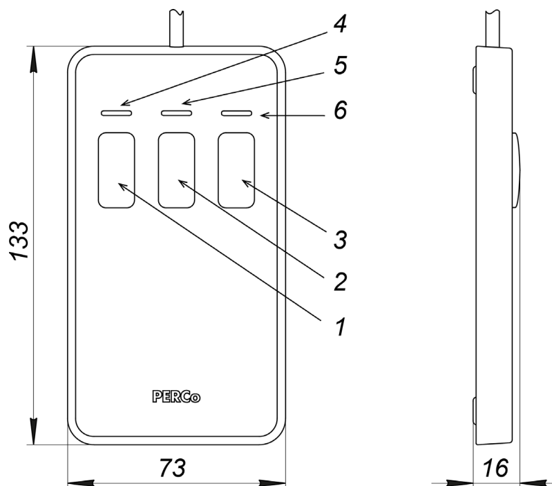
Рисунок 3. Общий вид и габаритные размеры ПДУ
