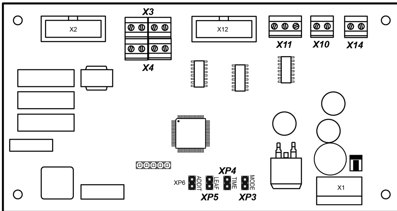
Рисунок 5. Расположение элементов на плате процессорного модуля
