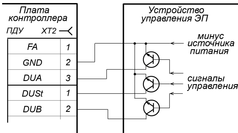
Рисунок 10. Управление ЭП схемой с открытым коллекторным выходом
