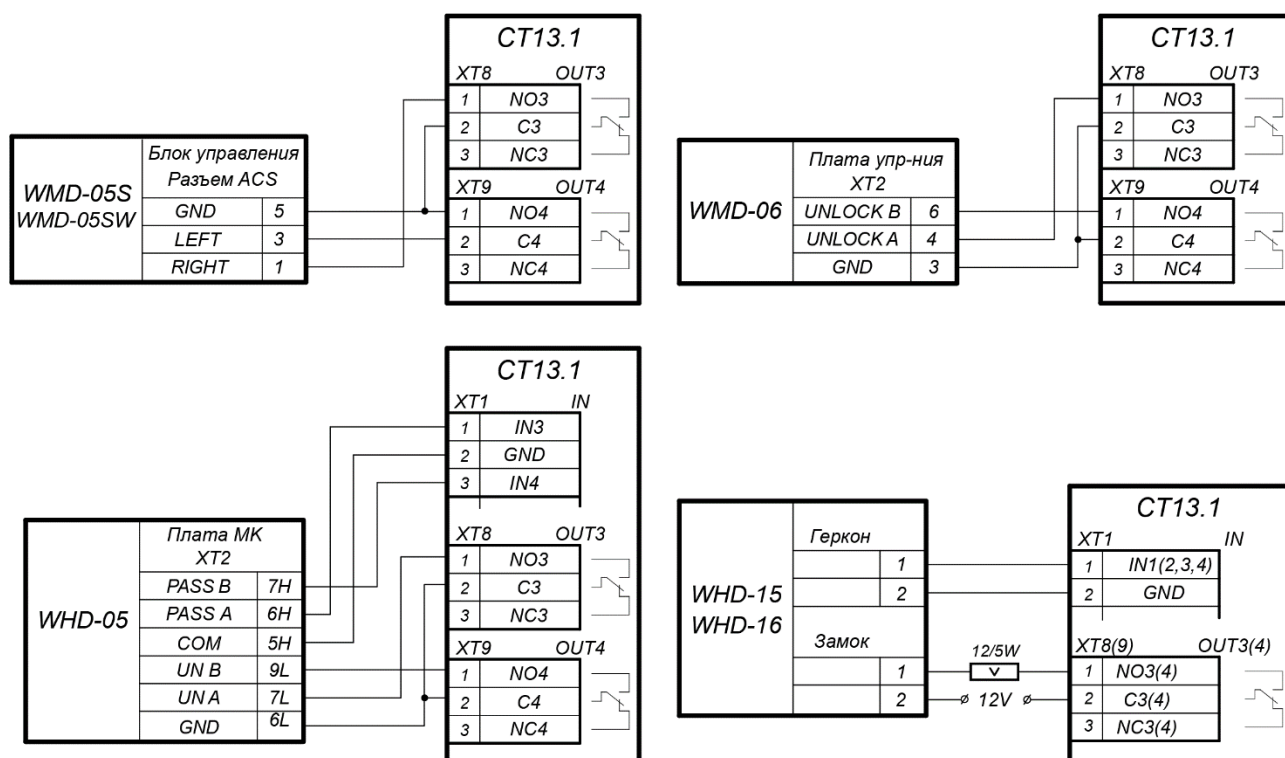
Рисунок 19. Схемы подключений калиток
