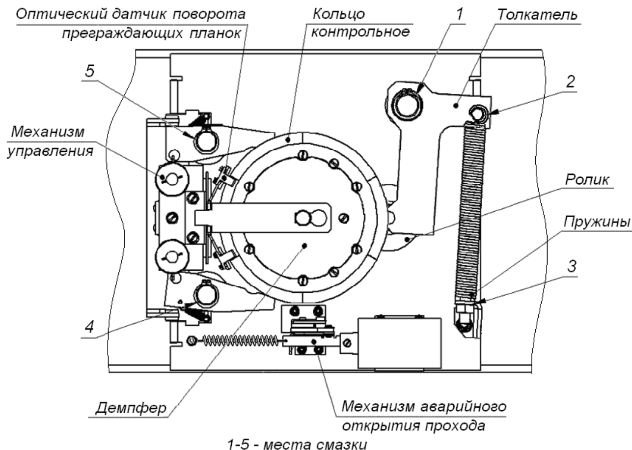
Рисунок 26. Расположение внутренних деталей и узлов стойки ЭП
