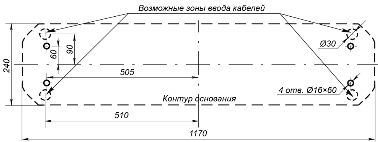
Рисунок 12. Схема разметки для установки стойки ЭП 1
