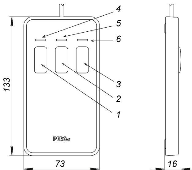
Рисунок 5. Общий вид и габаритные размеры ПДУ
