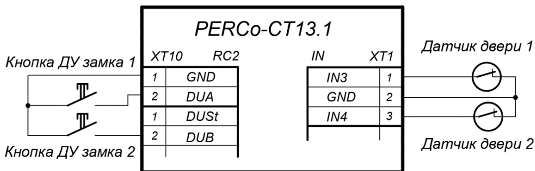
Рисунок 17. Схема подключений кнопок ДУ и датчиков двери
