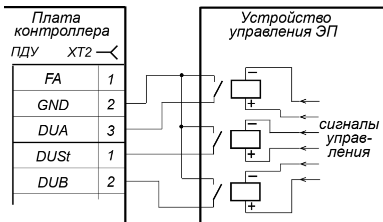
Рисунок 9. Управление ЭП нормально разомкнутым контактом реле
