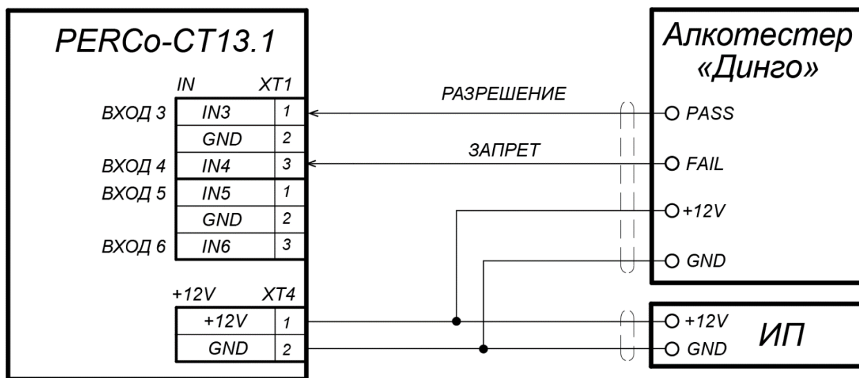
Рисунок 29. Схема подключения алкотестера «Динго В-02» (ООО СИМС-2)
