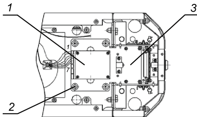
Рисунок 15. Механизм картоприемника
