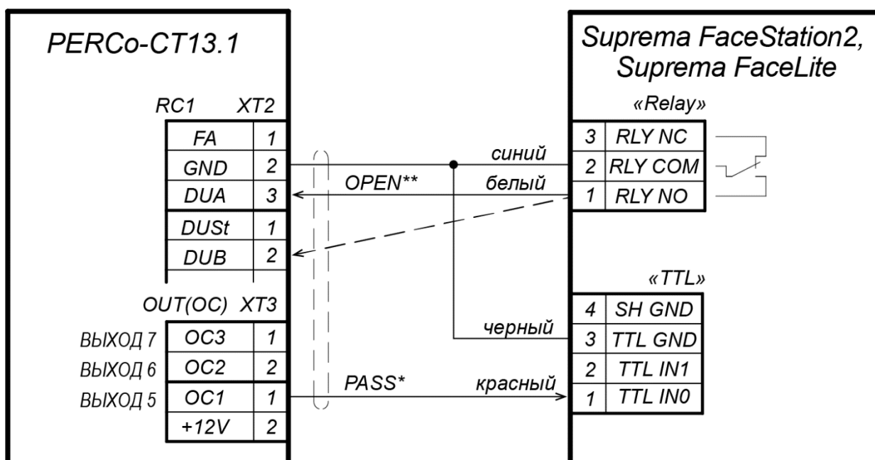
Рисунок 27. Схема подключения ТРЛ производства ZKTeco к контроллеру ЭП
