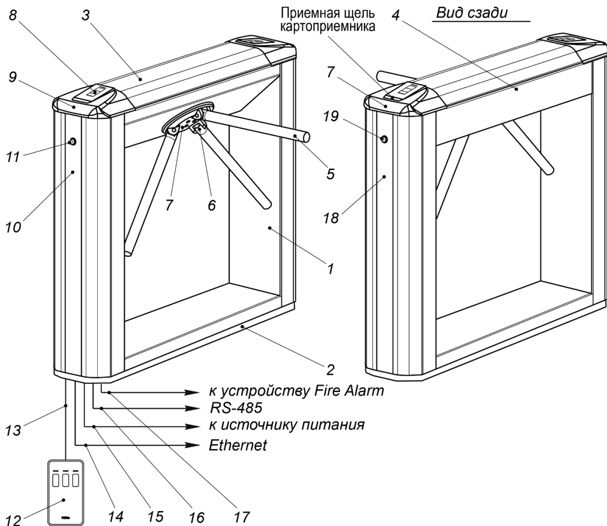
Рисунок 2. Устройство ЭП
