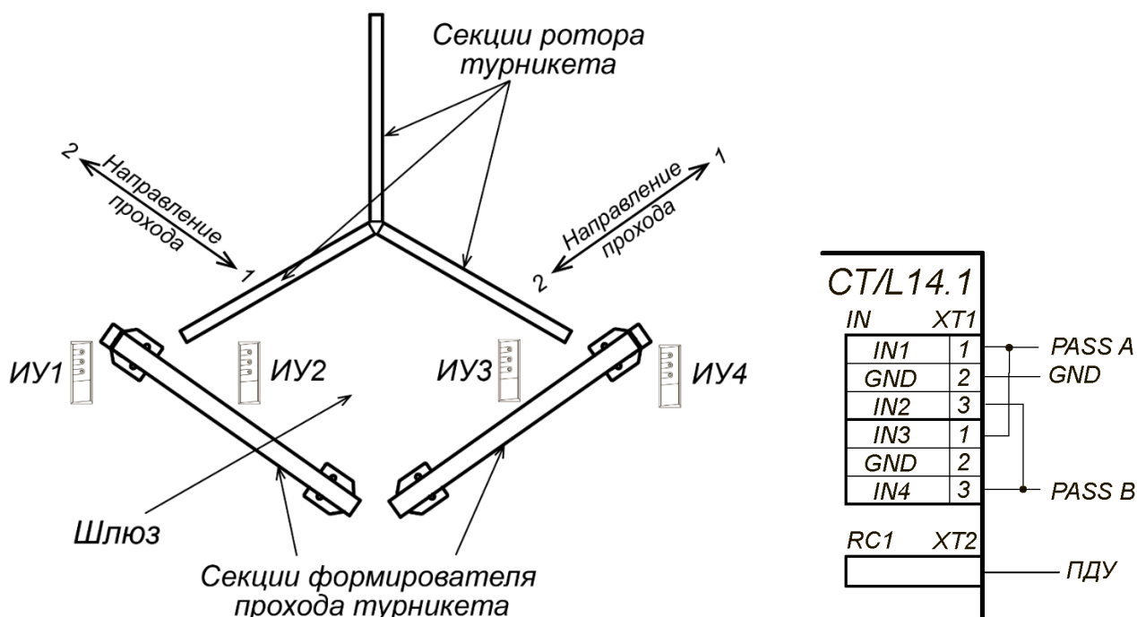
Рисунок 23. Схема шлюза из роторного турникета
