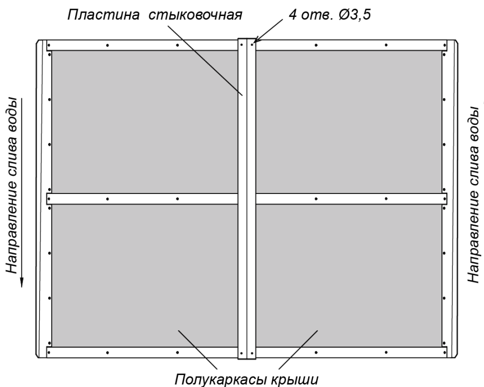
Рисунок 6. Вид сверху соединенных полукаркасов (1) и (2) с установленной стыковочной пластиной (6)
