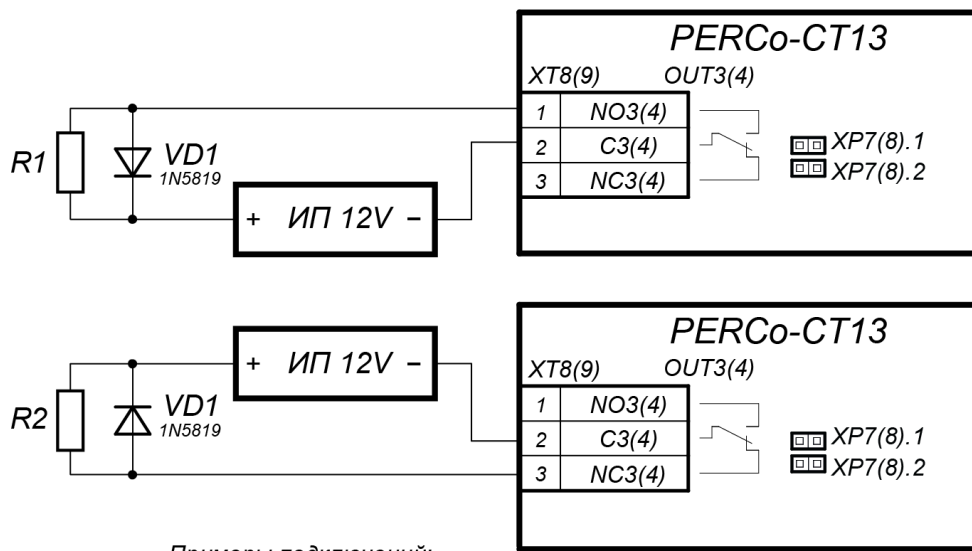
Рисунок 24. Схема подключений дополнительного оборудования к релейным выходам контроллера
