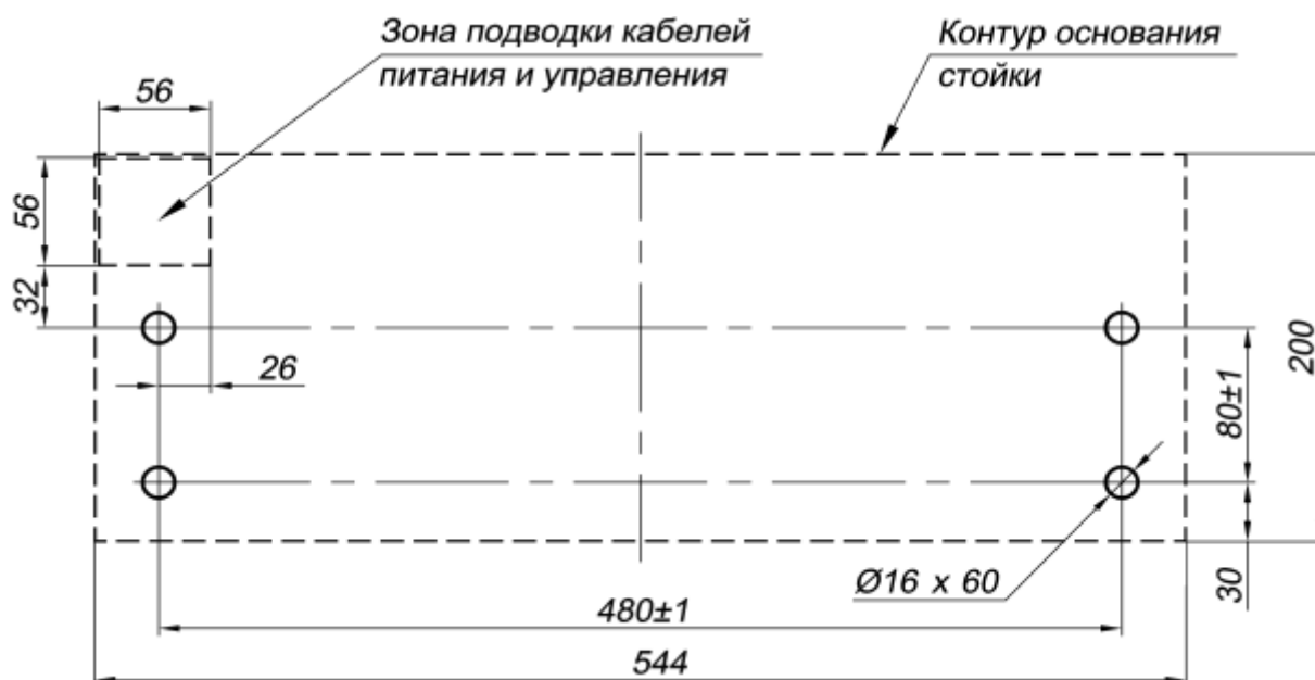
Рисунок 13. Схема разметки для установки стойки ЭП 1
