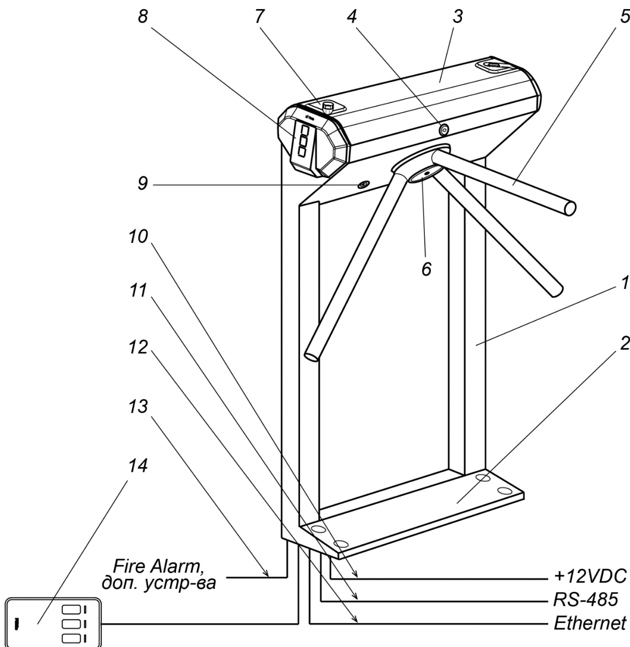
Рисунок 2. Устройство ЭП
