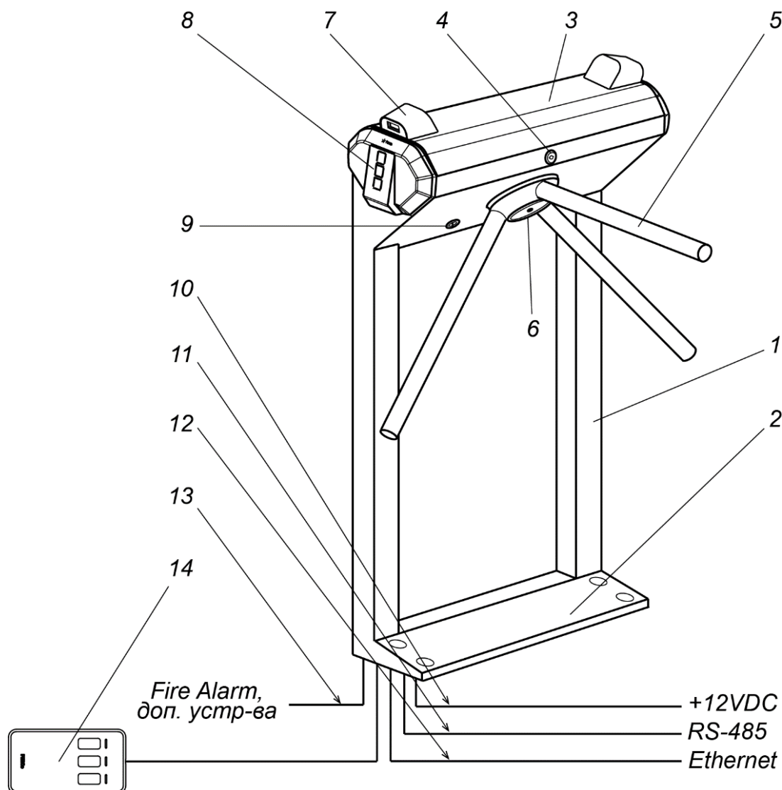
Рисунок 2. Устройство ЭП
