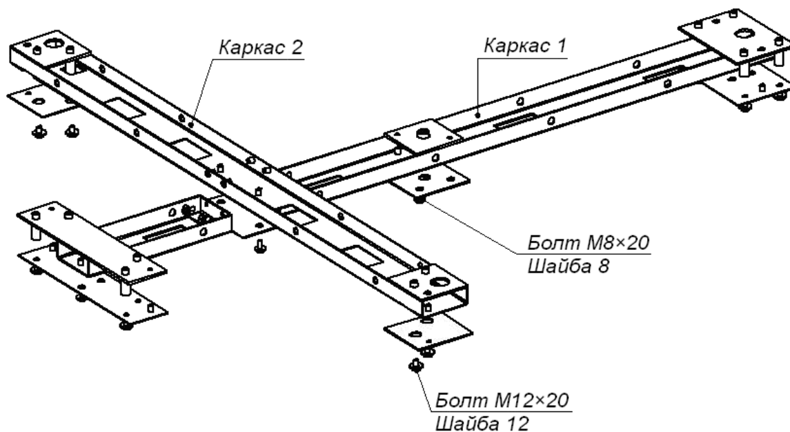
Рисунок 2 Схема сборки рамы. Шаг 1.
