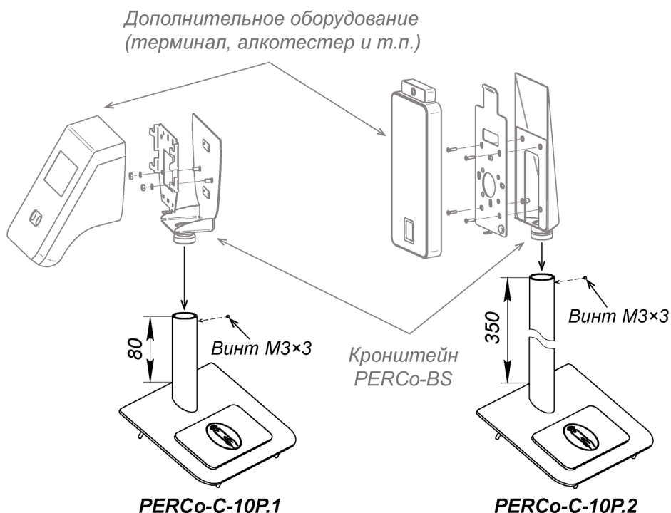
Рисунок 30. Внешний вид боковых крышек PERCo-C-10P.1 , PERCo-C-10P.2
