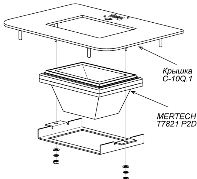
Рисунок 28. Боковая крышка PERCo-C-10Q.1 со сканером штрихкода Mertech T7821 P2D
