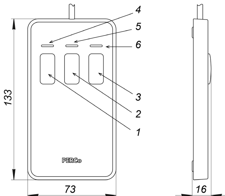
Рисунок 6. Общий вид и габаритные размеры ПДУ
