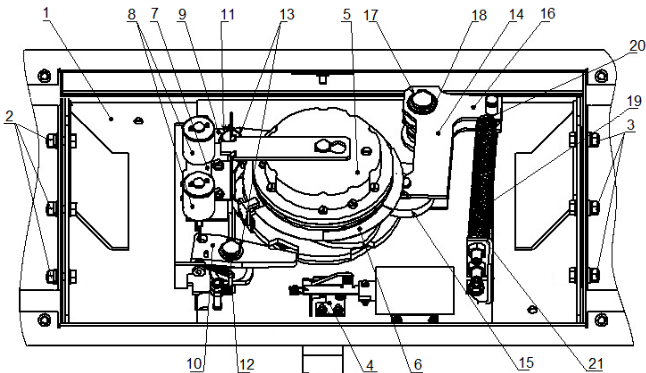
Рисунок 22. Узел вращения преграждающих планок турникета.
