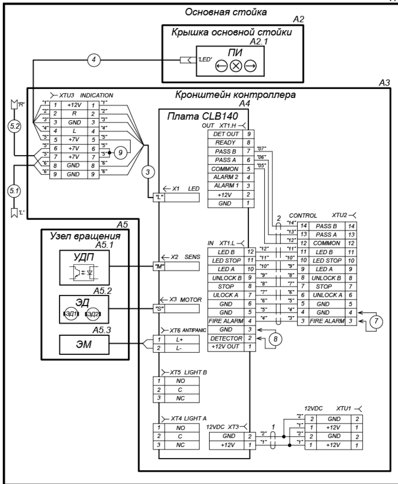
Рисунок 19. Схема внутренних соединений основной стойки
