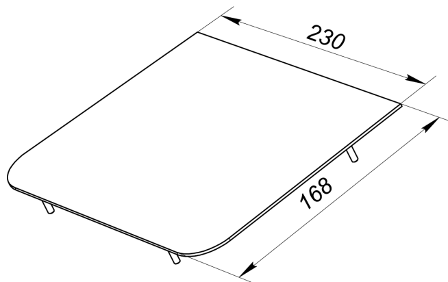
Рисунок 23. Габариты боковой крышки PERCo-C-10B
