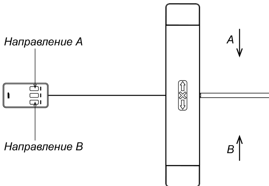
Рисунок 11. Стандартная ориентация ПДУ относительно стойки турникета
