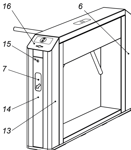
Рисунок 2. Устройство турникета PERCo-TTD-10A
