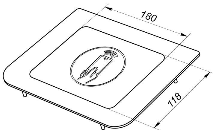
Рисунок 24. Внешний вид боковой крышки PERCo-C-10R
