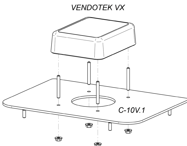
Рисунок 29. Боковая крышка PERCo-C-10V.1 с платежным терминалом Vendotek VX
