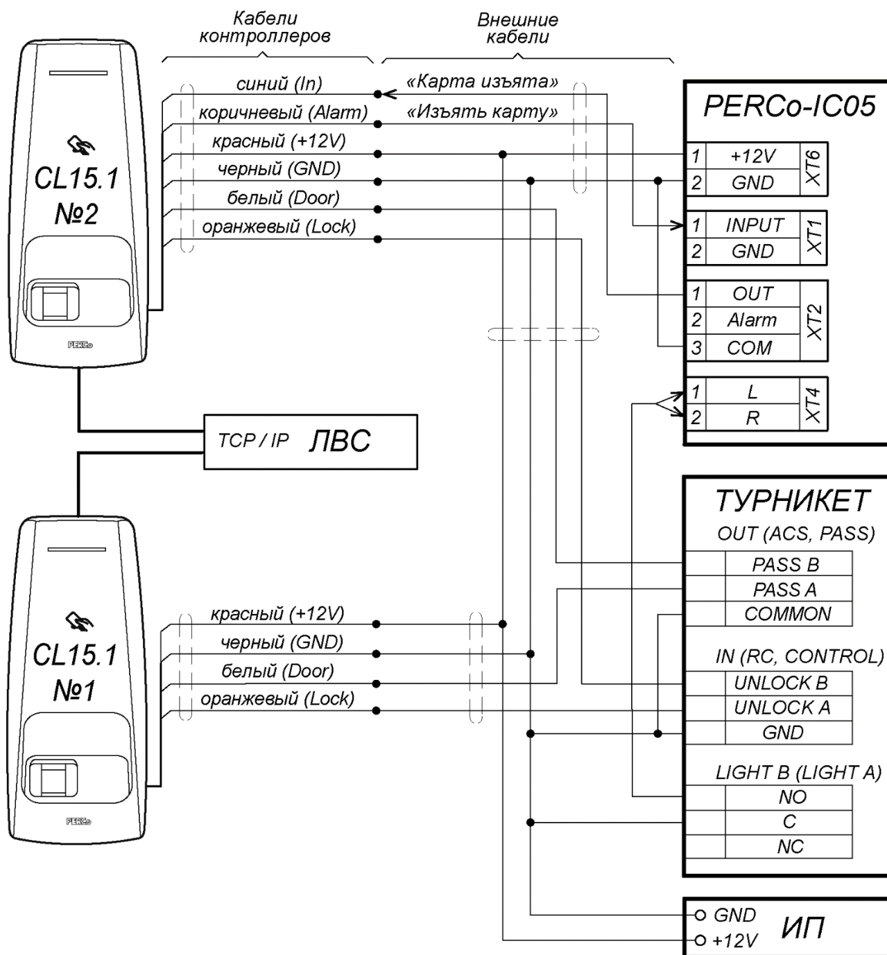
Рисунок 13. Схема подключения PERCo-CL15.1 к турникету с картоприемником PERCo-IC05
