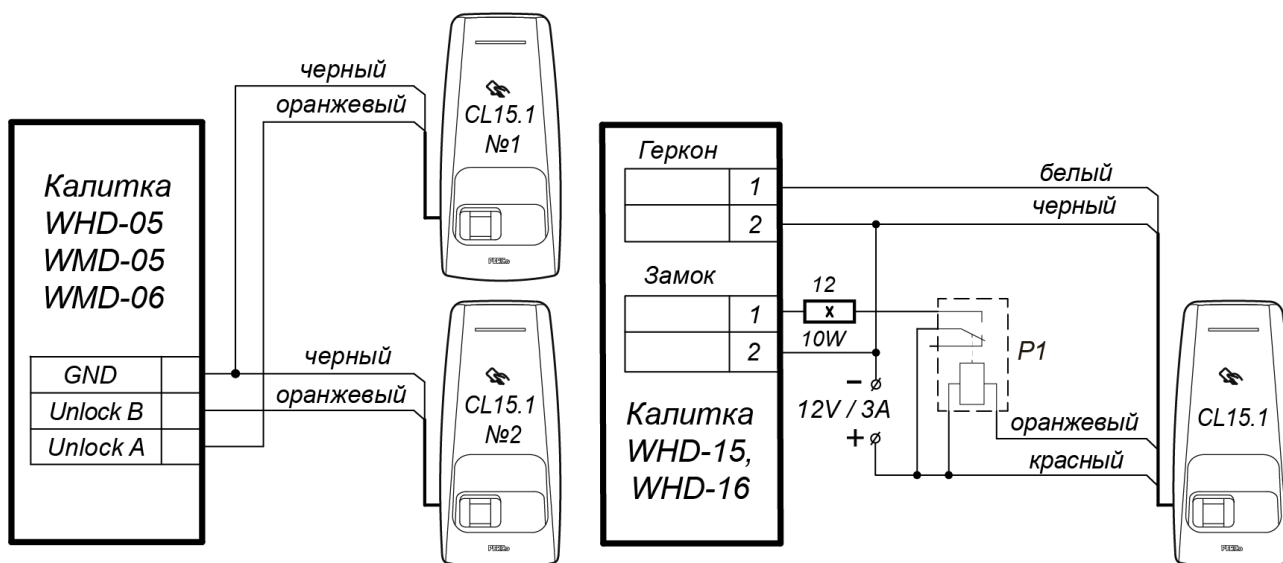
Рисунок 8. Схемы подключений калиток
