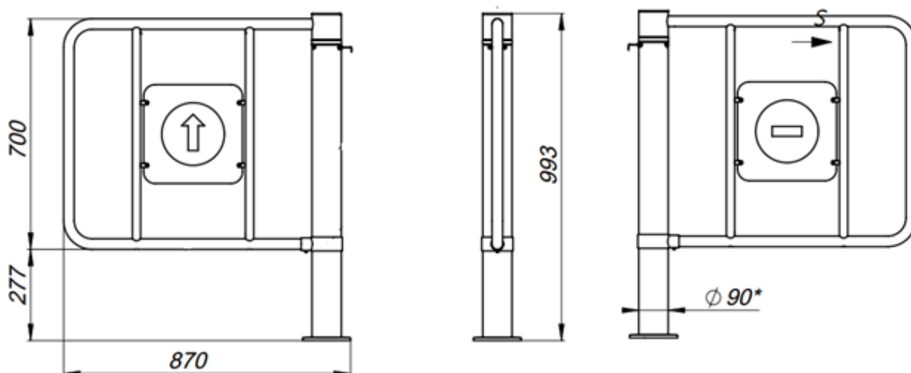
Рисунок 2 – Габаритные размеры калитки размером 870 мм
