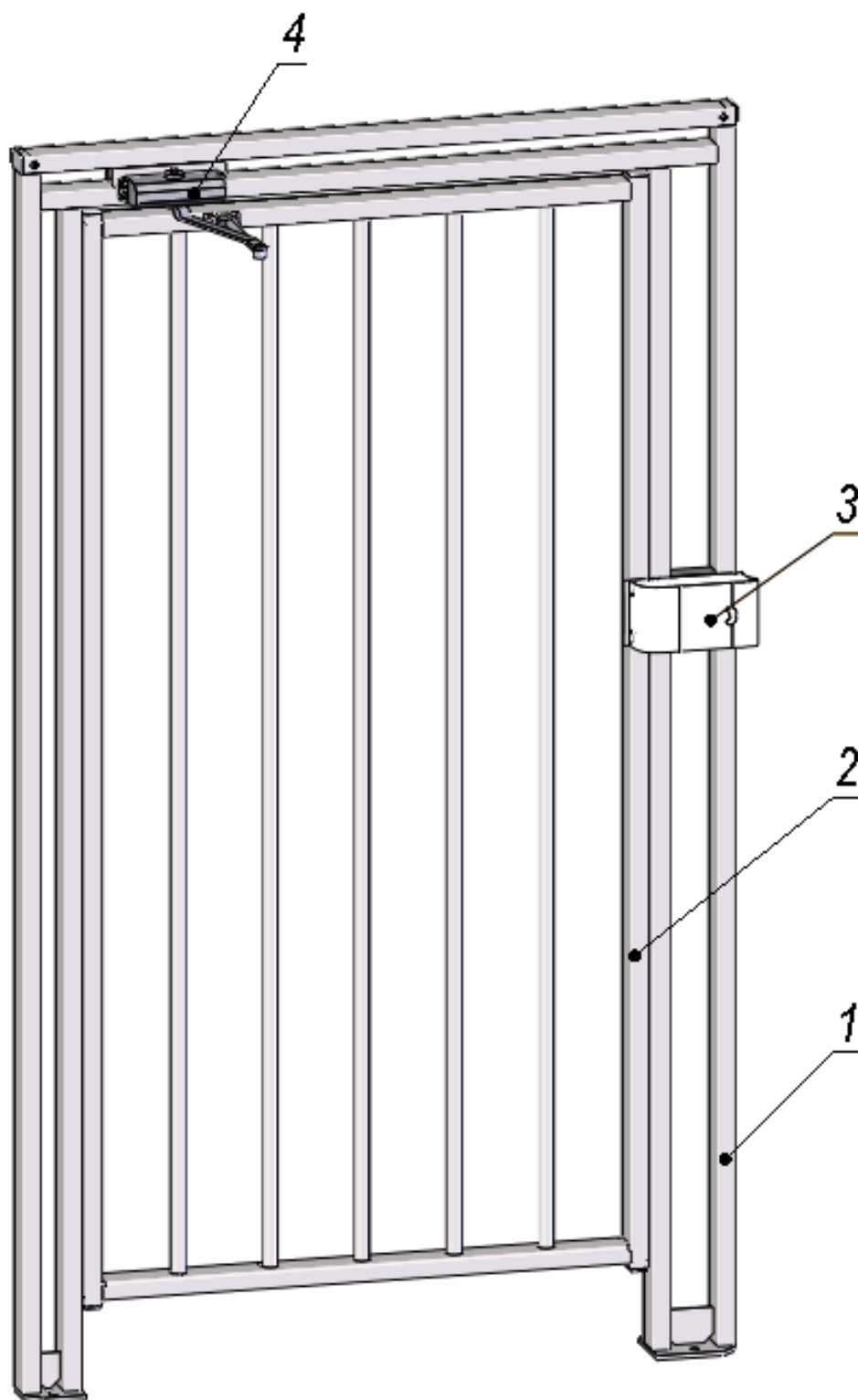
Рисунок 2. Общий вид калитки
