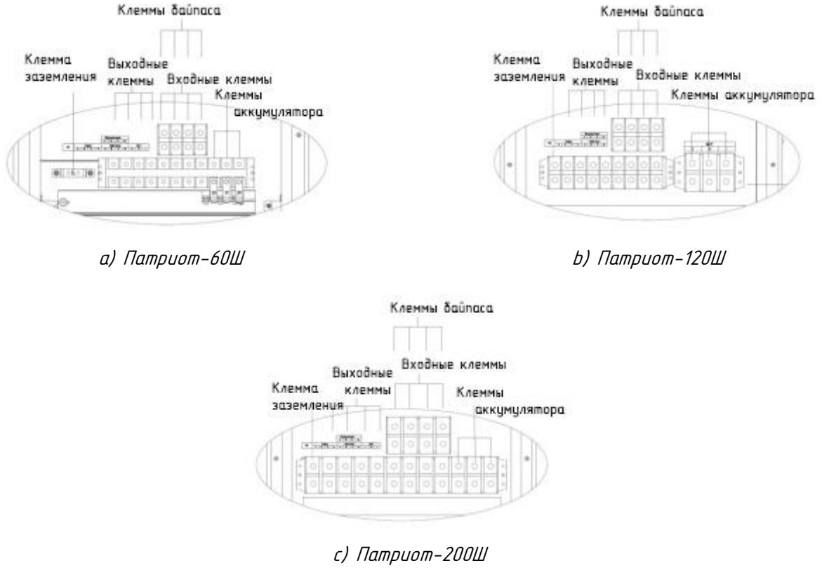
Рис. 1-27 Подключение ИБП к сети питания
