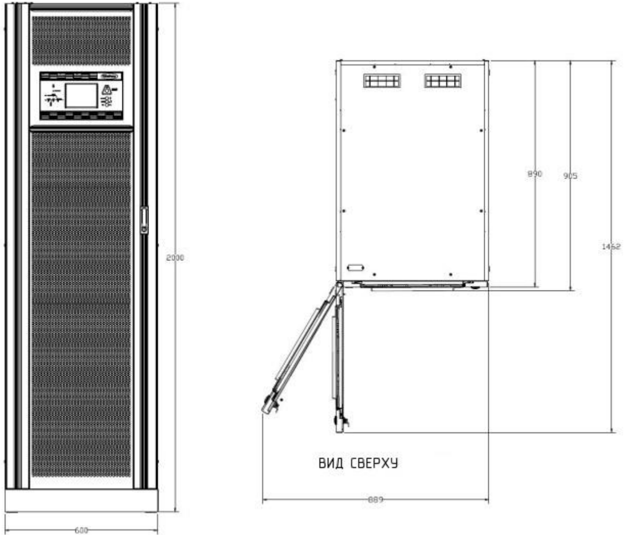
Рис. 1-26с Внешние габариты ИБП Патриот-200Ш
