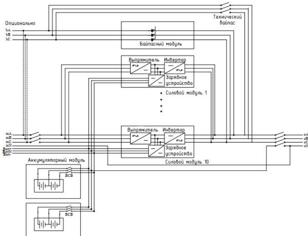
Рис. 2-1 Однолинейная схема
