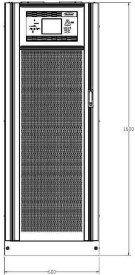
Рис. 1-26а Внешние габариты ИБП Патриот-60Ш Рис. 1-26б Внешние габариты ИБП Патриот-120Ш
