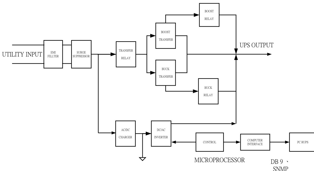
Рис.3.1-1 Блок-схема ИБП серии Monolith K 1к - 3к
