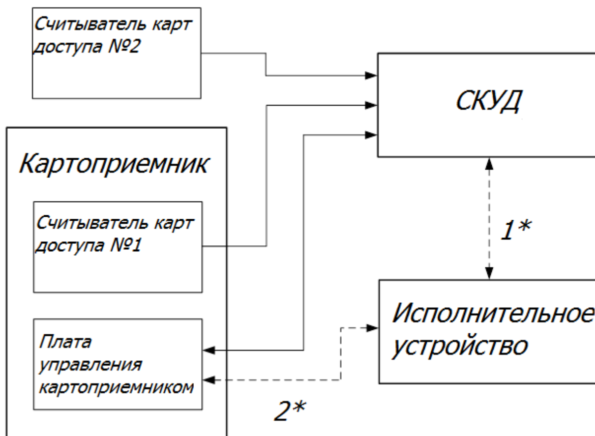
Рисунок 13 - Структурная схема №1
