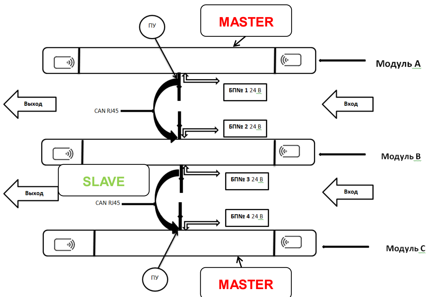
Рисунок 9 - Схема подключения модулей турникета
