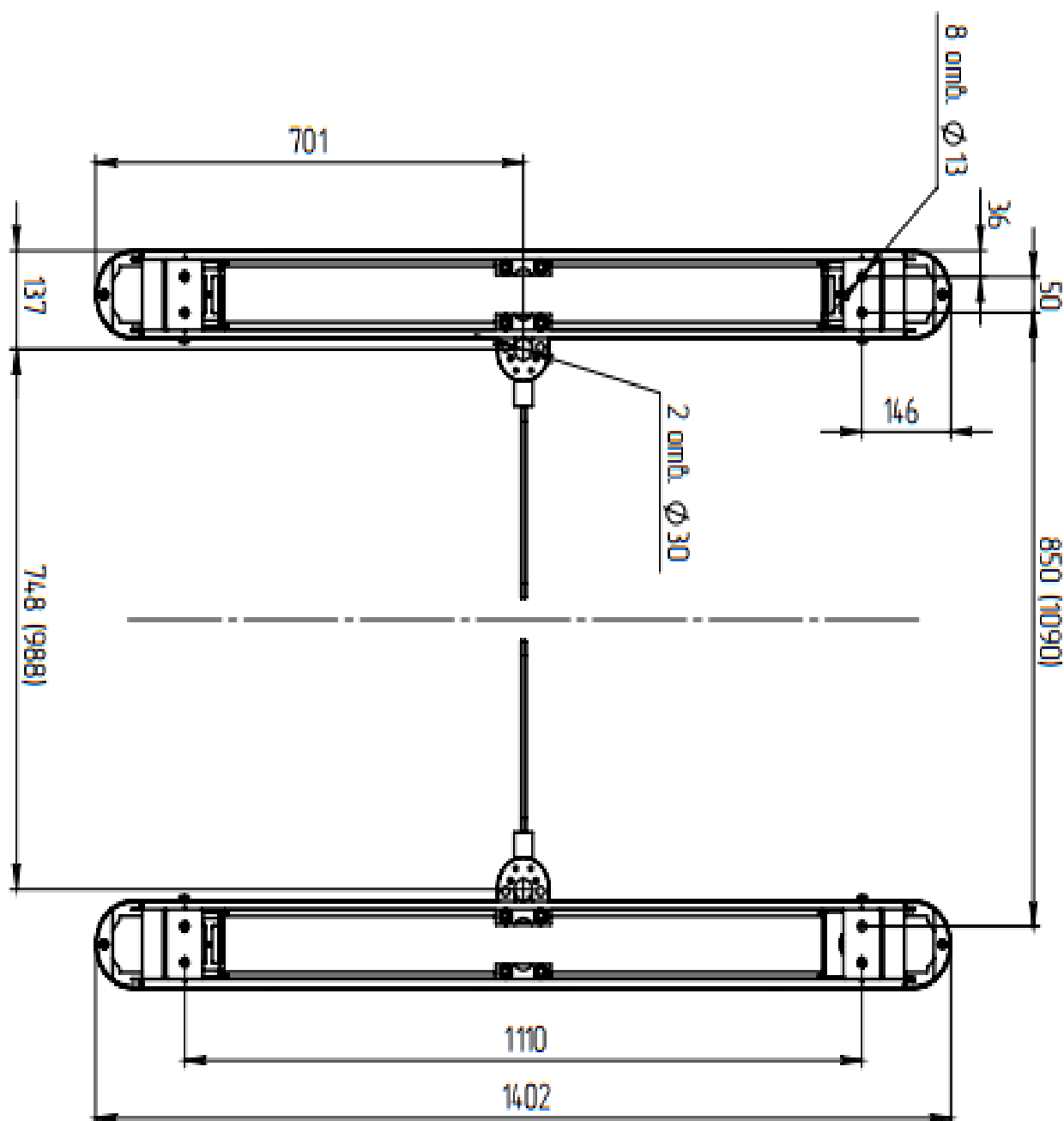
Рисунок 2 – Установочные размеры площадки турникета при ширине прохода 660 мм
