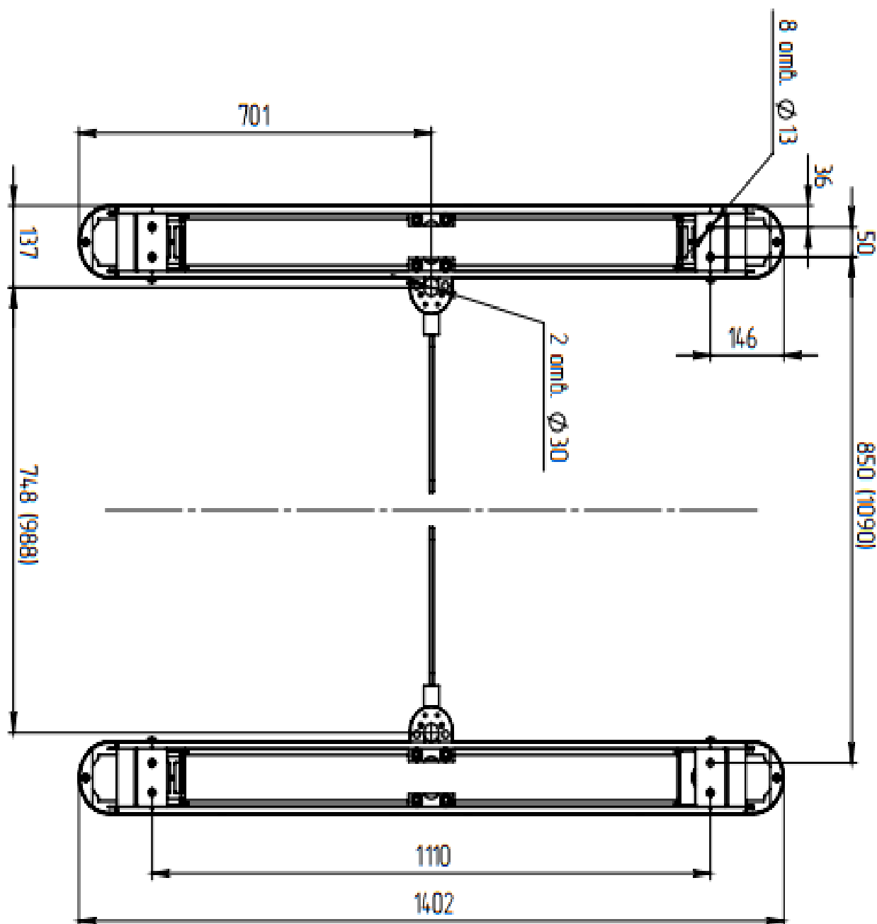
Рисунок 12 - Расположение монтажных отверстий относительно внешних габаритов турникета.
