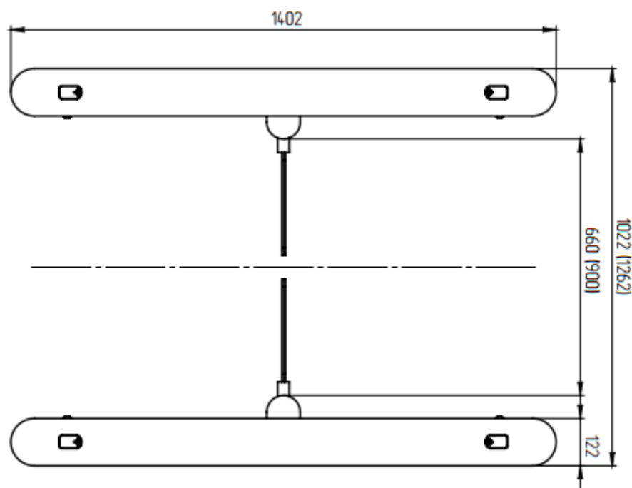
Рисунок 1 – Габаритные размеры турникета
