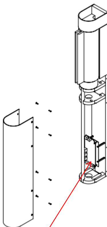
материнская плата
