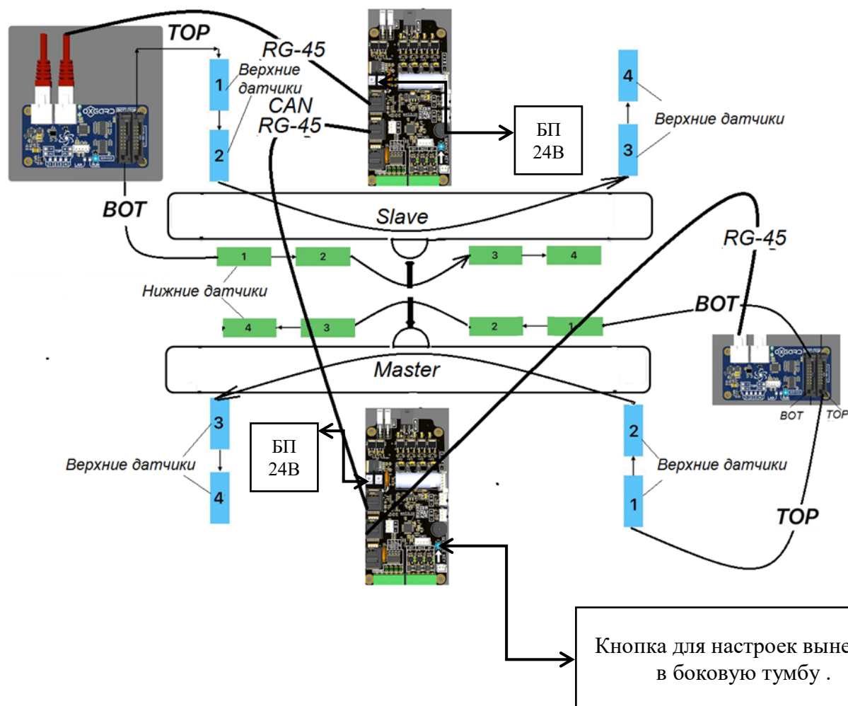
Рисунок 5 – Схема соединений датчиков модулей
