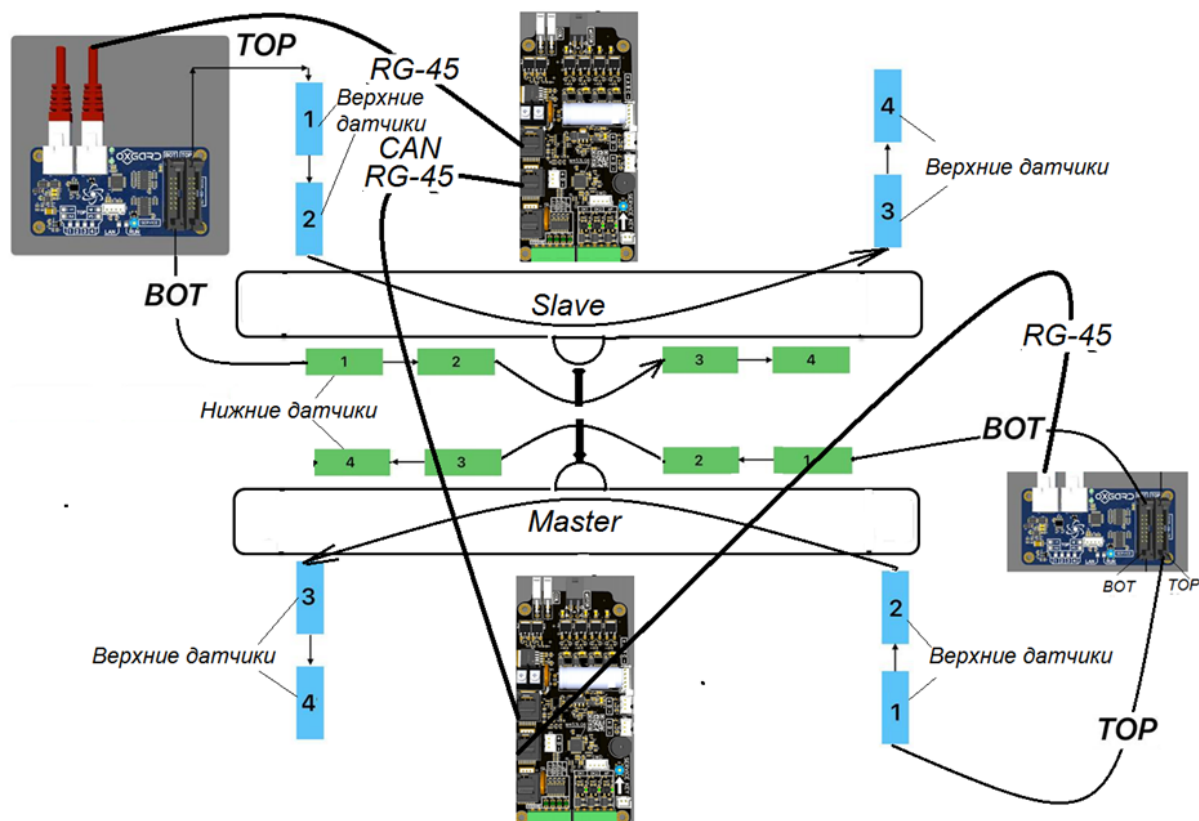
Рисунок 15-Схема минимальных подключений для синхронной работы створок турникета
