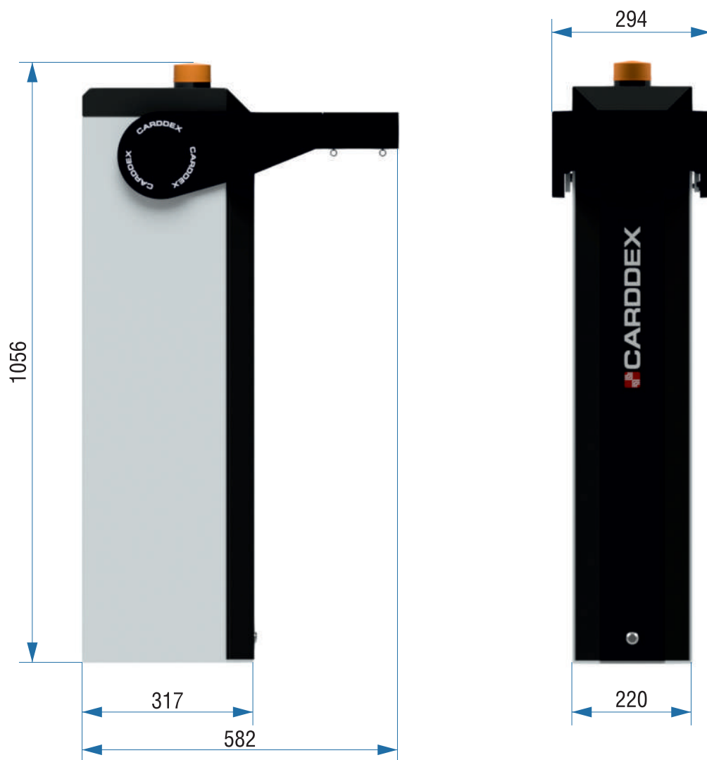
Рисунок 5.1 Габаритные размеры шлагбаума
