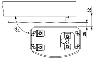
Малюнок 4. Розташування монтажної основи відносно до стулки
