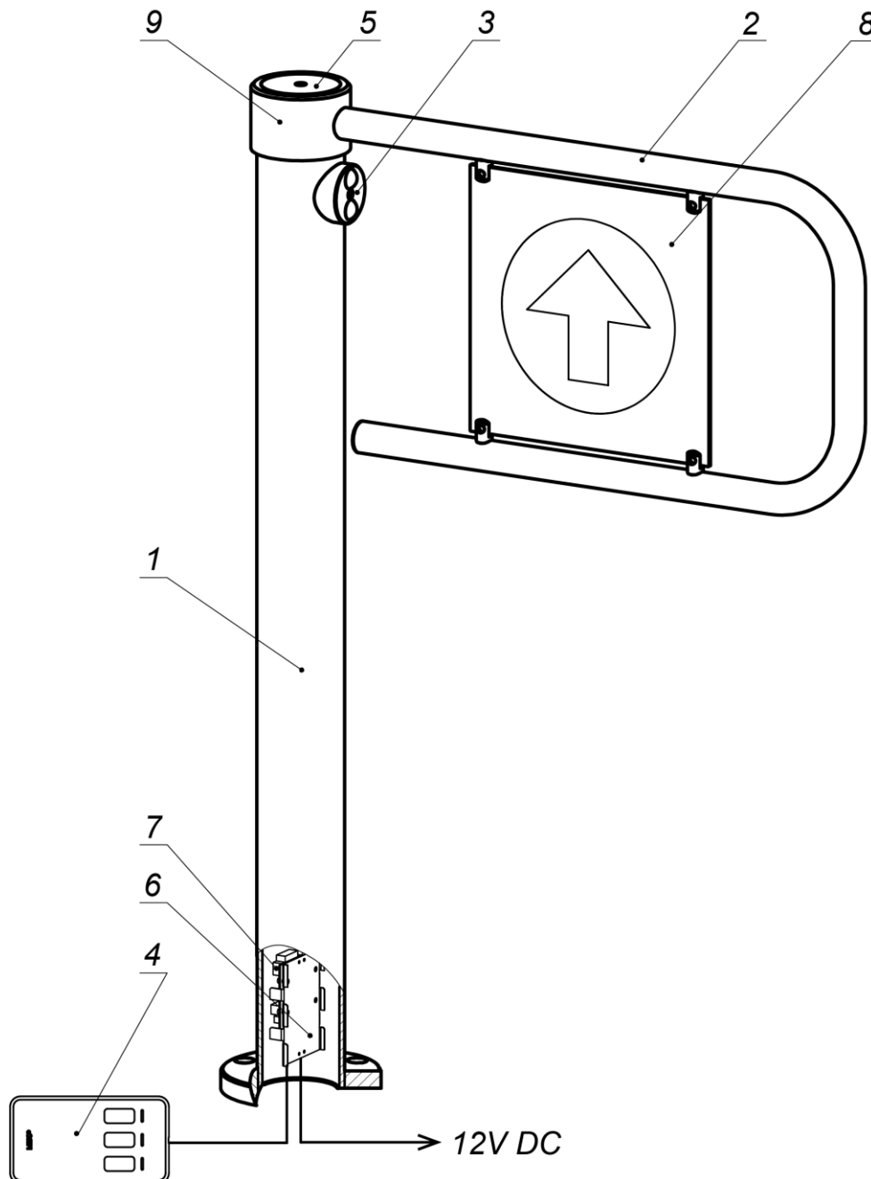
Рисунок 2. Общий вид калитки:
