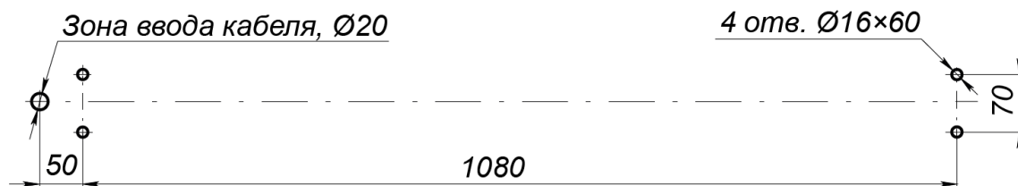
Рисунок 3. Схема разметки для установки калитки 1
