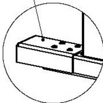
рис. 5 Установка накладак PERCo-RF01 0-07
